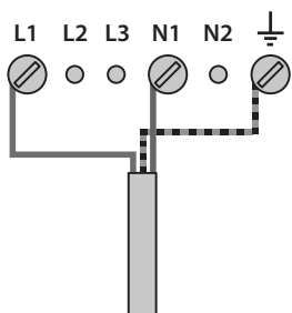
2 - Burner 1x 230 V
