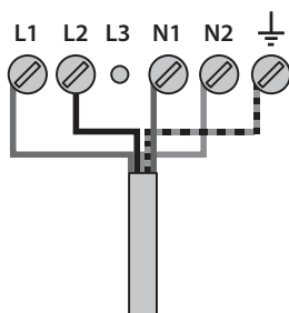
4 - Burner 1x 230 V
