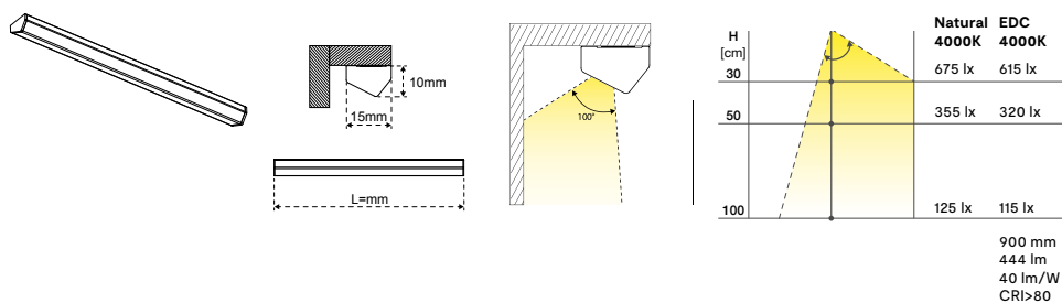
| Regleta Kea SIN interruptor (instalación delantera)
