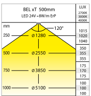
BELLxT con sensor PIR
