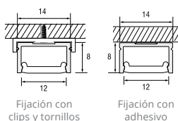
Clips de fijación
