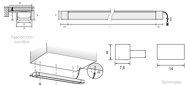
Fijación mediante tornillos
