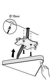
Detalle de la fijación oculta
