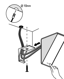
Detalle de la fijación oculta
