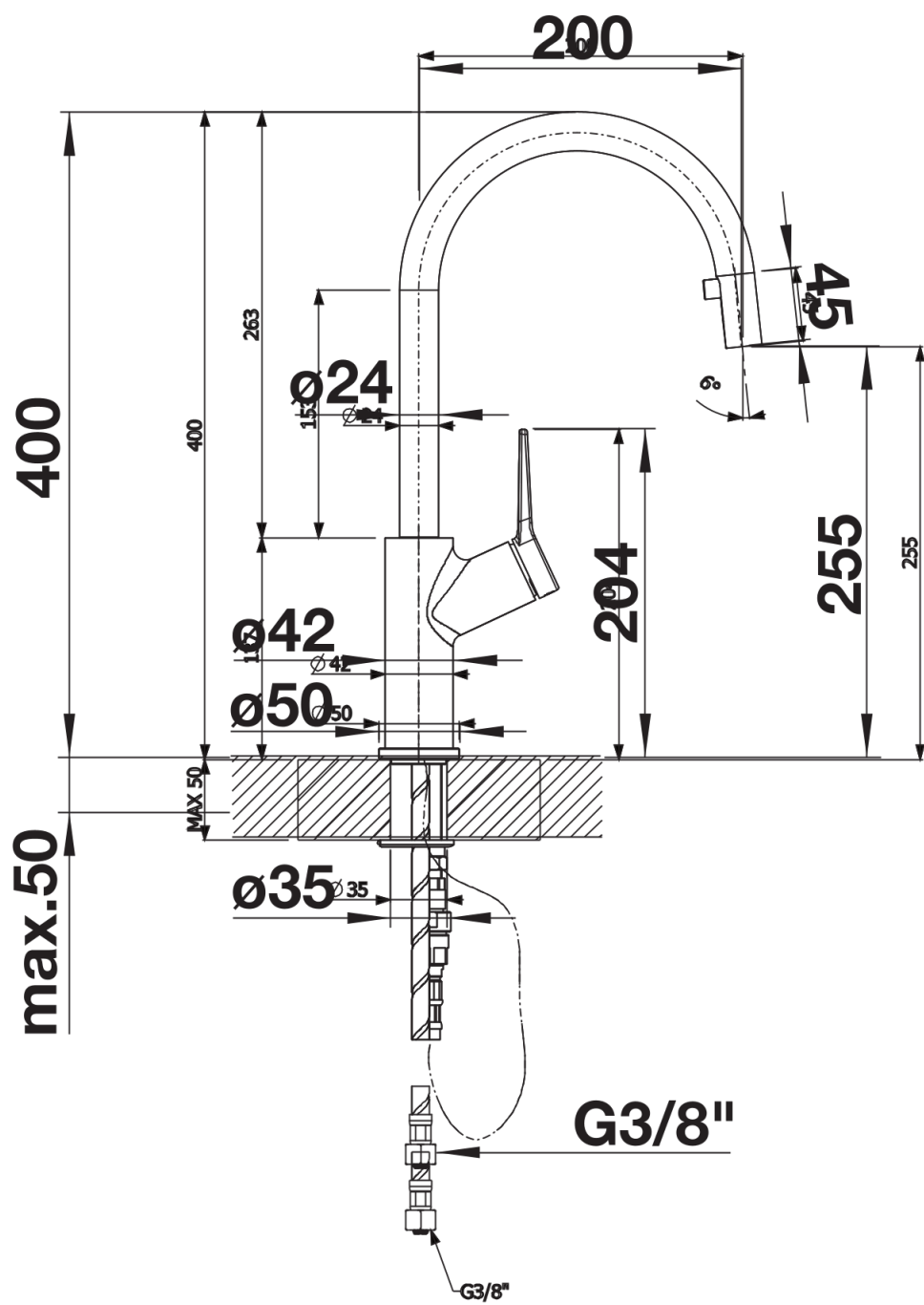
Vista lateral
