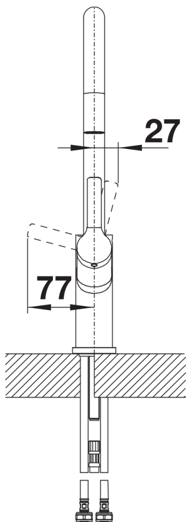
Vista lateral da mudança manual 2D
